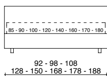
BASE CONTENITORE A 1 APERTURA O A 2 POSIZIONI SINGLE-OPENING OR DUAL-POSITION STORAGE BASE
