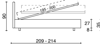
BASE CONTENITORE A 1 APERTURA O A 2 POSIZIONI SINGLE-OPENING OR DUAL-POSITION STORAGE BASE
