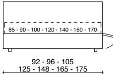
FASCIA APRIBILE DX - SX PER INSERIMENTO 2° LETTO ESTRAIBILE O CASSETTONI L-R OPENABLE BED SURROUND FOR FITTING A 2ND PULL-OUT BED OR STORAGE DRAWERS
