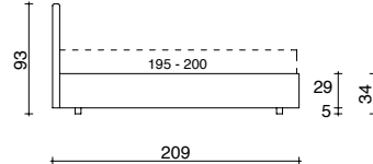
FASCIA APRIBILE DX - SX PER INSERIMENTO 2° LETTO ESTRAIBILE O CASSETTONI L-R OPENABLE BED SURROUND FOR FITTING A 2ND PULL-OUT BED OR STORAGE DRAWERS
