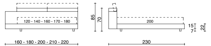
SPONDA LATERALE SX - DX TESTATA CON MECCANISMO FASCE IMBOTTITE H. 15 CM SIDE FRAME L-R HEADBOARD WITH MECHANISM, PADDED SURROUND H. 15 CM
