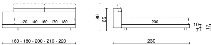
SPONDA LATERALE SX - DX TESTATA CON MECCANISMO FASCE IMBOTTITE H. 10 CM SIDE FRAME L-R HEADBOARD WITH MECHANISM, PADDED SURROUND H. 10 CM
