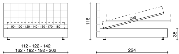
SPONDA LARGE ALTO TESTATA TRAPUNTATA H. 116 CM BASE CONTENITORE A 1 APERTURA O A 2 POSIZIONI LARGE FRAME TALL QUILTED HEADBOARD H. 116 CM, SINGLE-OPENING OR DUAL-POSITION STORAGE BASE
