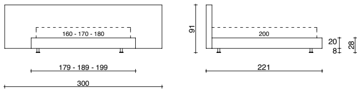
LONG SPONDA LARGE H. 91 CM FASCE IMBOTTITE H. 20 CM LONG FRAME LARGE H. 91 CM, PADDED SURROUND H. 20 CM
