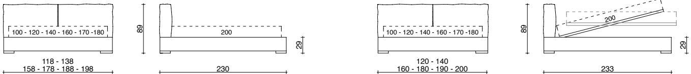
BASE CONTENITORE A 1 APERTURA O A 2 POSIZIONI SINGLE-OPENING OR DUAL-POSITION STORAGE BASE
