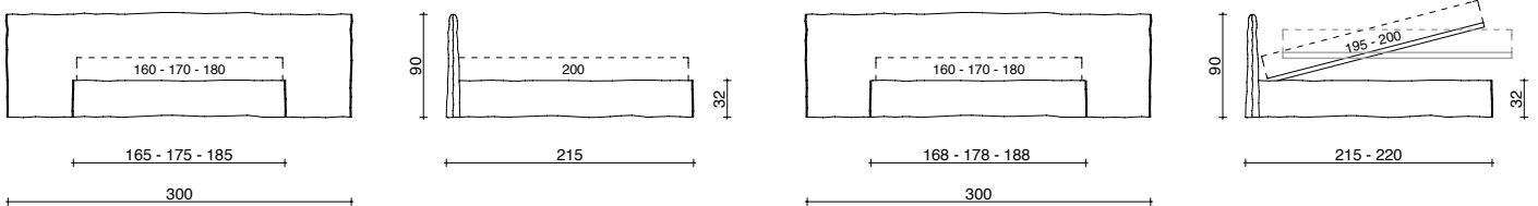
BASE CONTENITORE A 1 APERTURA O A 2 POSIZIONI SINGLE-OPENING OR DUAL POSITIONS STORAGE BASE
